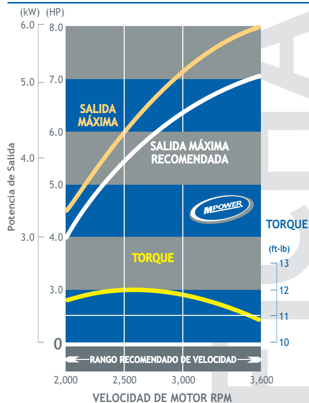
CURVA DE DESEMPEÑO MP-8
